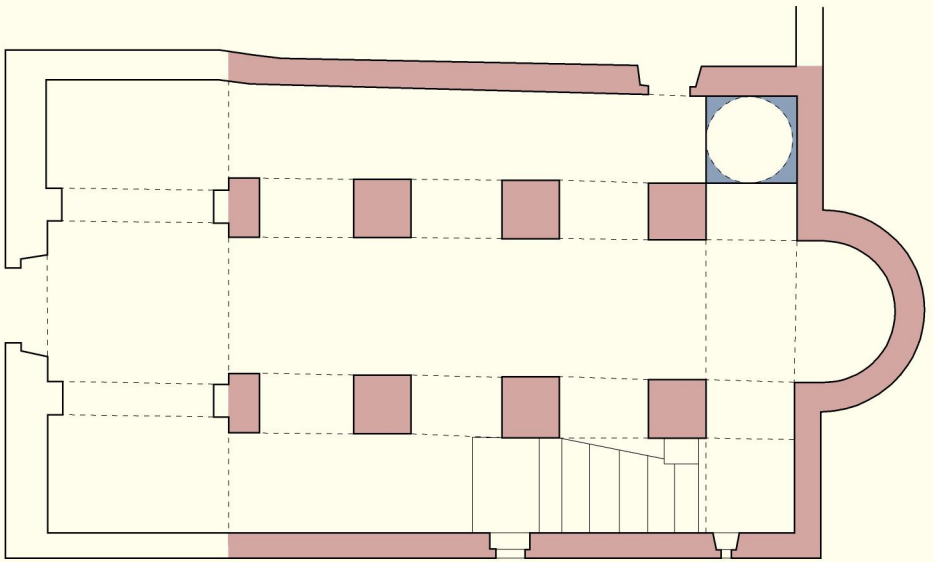
Pianta
