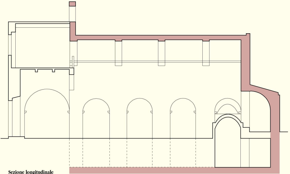
Sezione longitudinale
