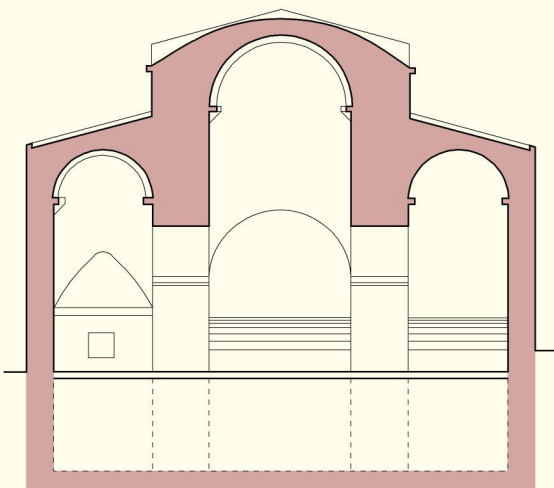
Sezione trasversale
